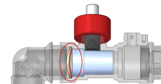
Utbytt nippel: Böjd packning för att hålla turbinen i korrekt läge.
