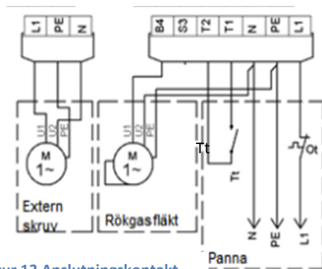
Figur 13 Anslutningskontakt
