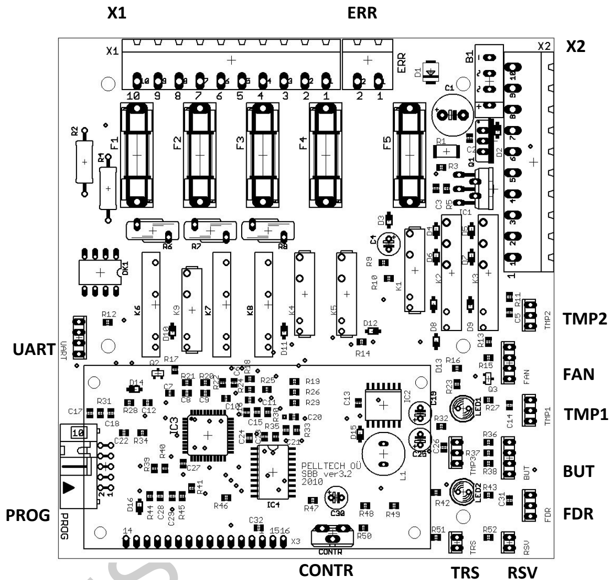
Figur 23 Kretskort SBB 3.2
