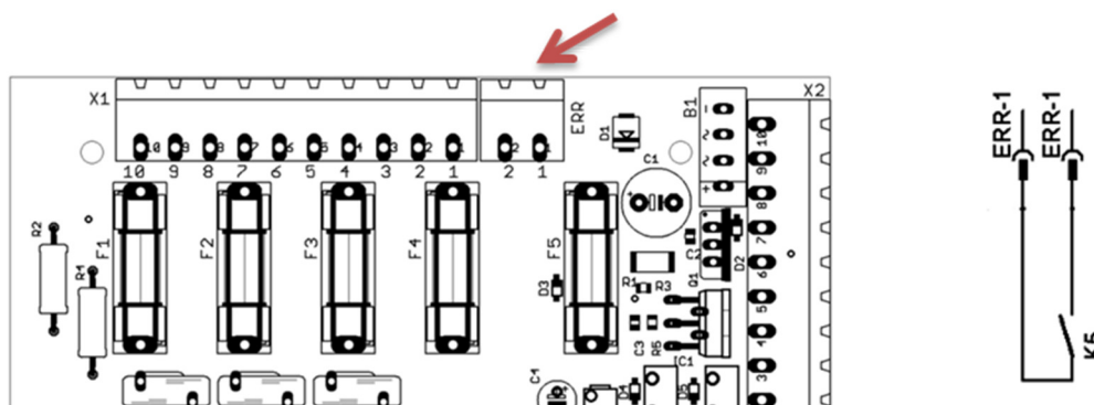
Figur 17 Larmutgång
