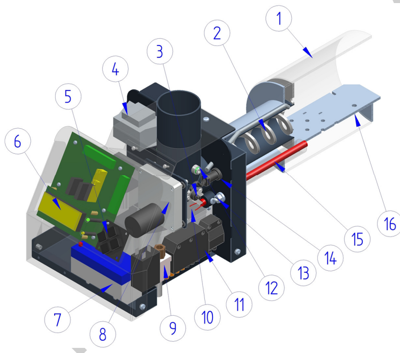
Figur 1 Brännarens huvudkomponenter
