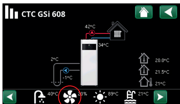
Menu "Driftsinfo".
