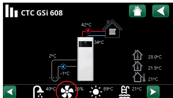
Valikko "Käyttötiedot".
