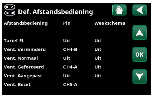
Menu "Installateur/Definieer/Afstandsbediening".
