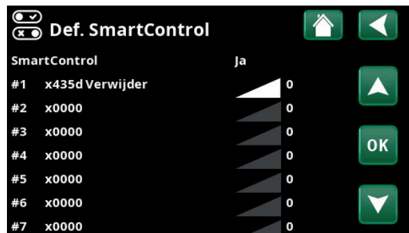
Menu "Installateur/Definieer/SmartControl".
