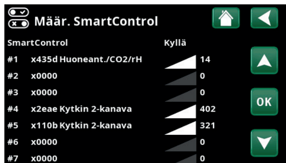
Valikko "Edistyneempi/Määrittele/SmartControl".
