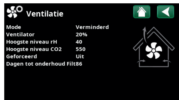
Menu "Werking/Ventilatie".
