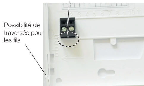
Plaque de base : connexion, fils d'alimentation
