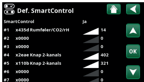
Menu "Avanceret/Definere/SmartControl".
