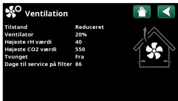
Menu "Driftsinfo/Ventilation".
