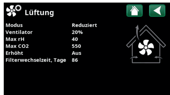
Menü „Betrieb/Lüftung“.
