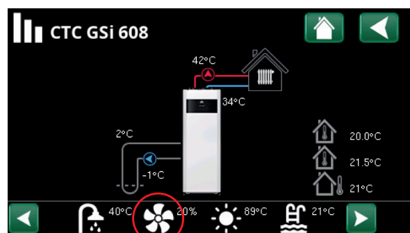
Menu "Werking".
