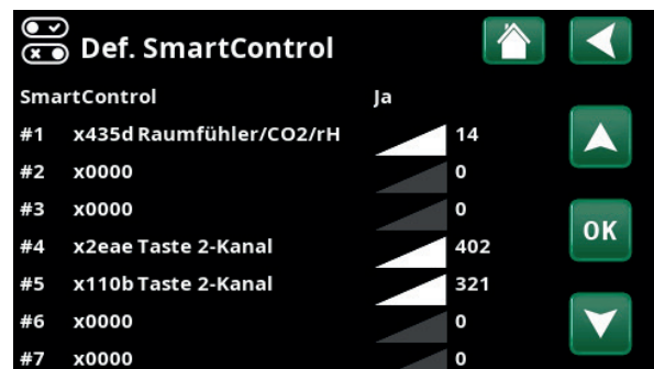
Menü „Fachmann/System/SmartControl“.
