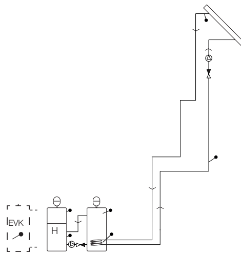
Sol: Alternativ solslinga
