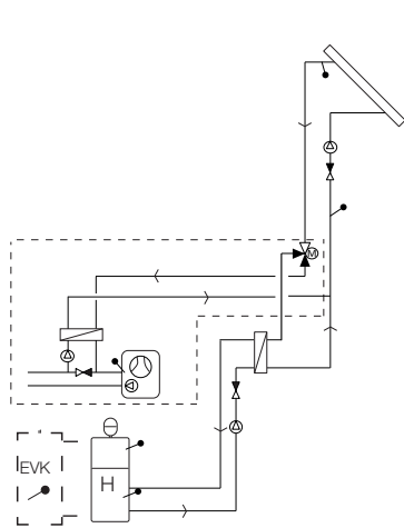
Sol: Option värma borrhål
