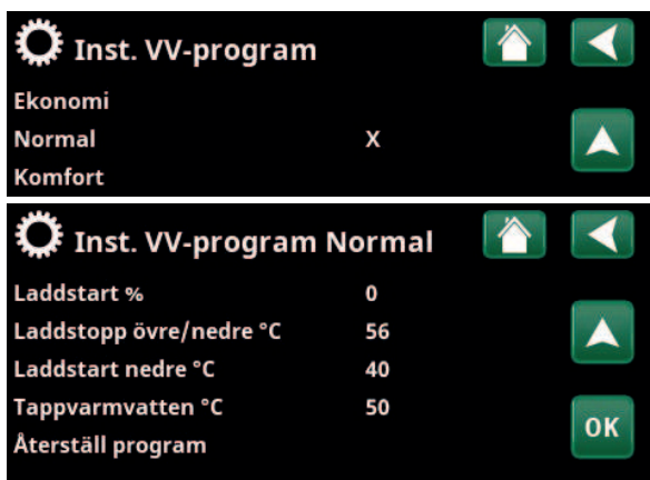
Menyer "Avancerat/Inställningar/Varmvatten/VV-program".
