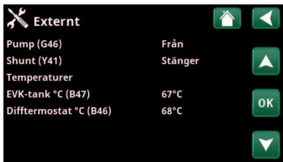
Meny "Avancerat/Service/Funktionstest/Difftermostat".
