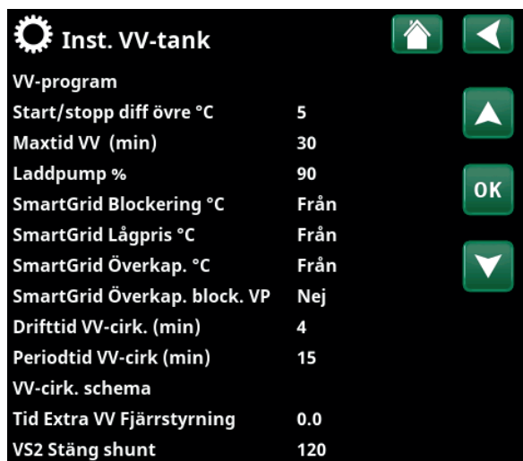
Meny "Avancerat/Inställningar/Varmvatten".
