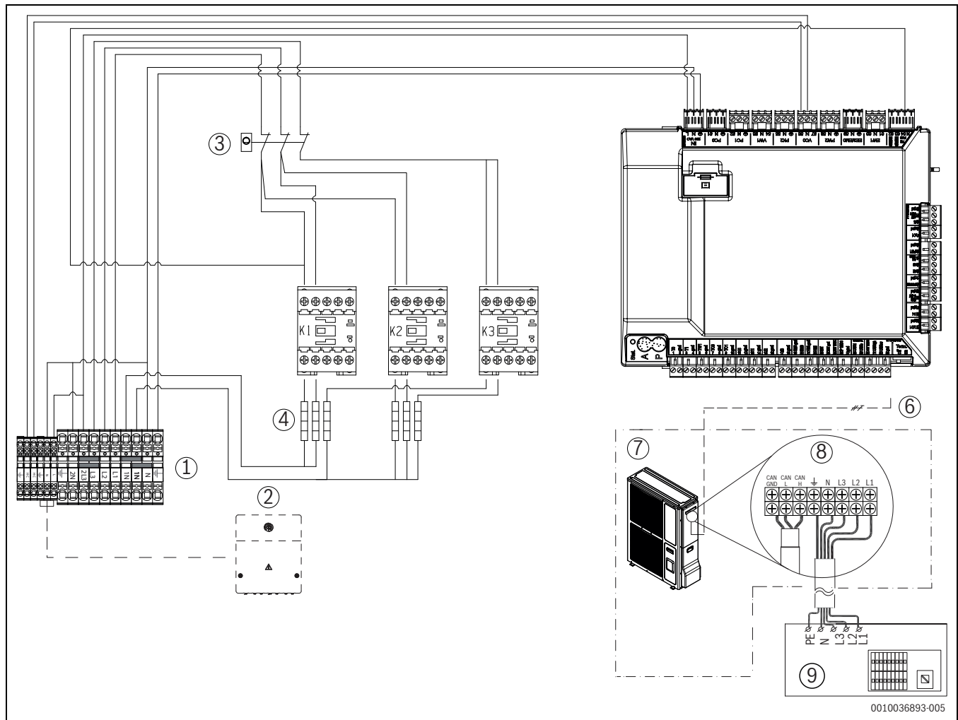
Bild 37 Inneenhet på 400 V 3 N~ med uteenhet på 400 V 3 N~
