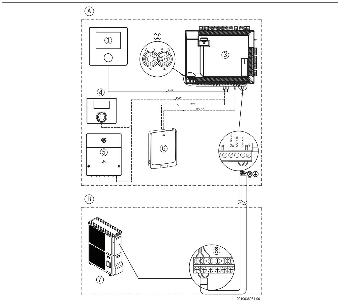
Bild 32 CAN- och EMS-anslutningar
