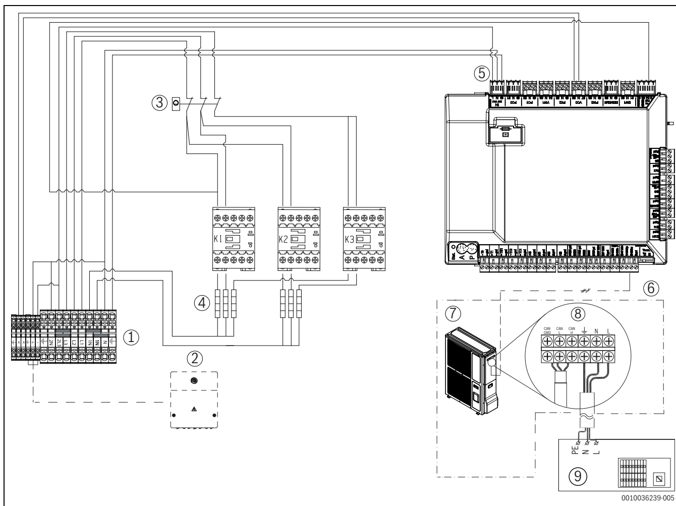
Bild 36 Inneenhet på 400 V 3 N~ med uteenhet på 230 V~
