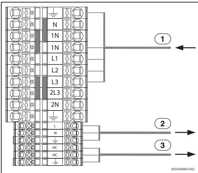
Bild 15 Anslutningsplintar för elanslutning, 9 kW 400 V 3 N~
