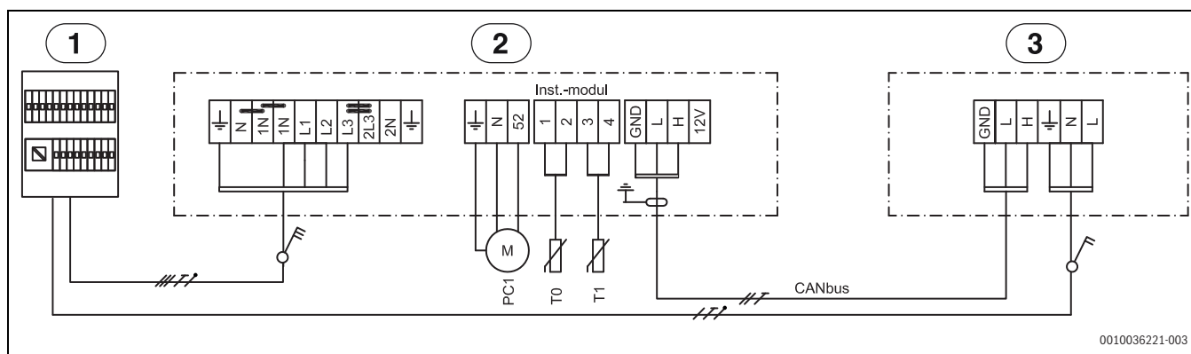
Bild 34 Anslutningsschema 9kW 3N~
