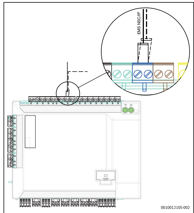
Bild 20 EMS anslutning på Installermodul
