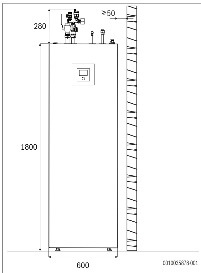
Bild 5 Mått (mm)
