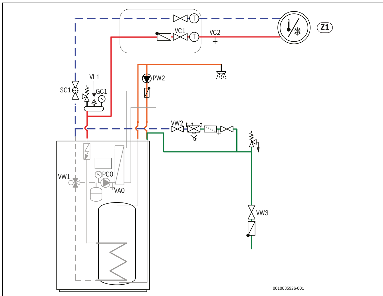
Bild 16 Ventilera inneenheten med ett integrerat eltilfskott
