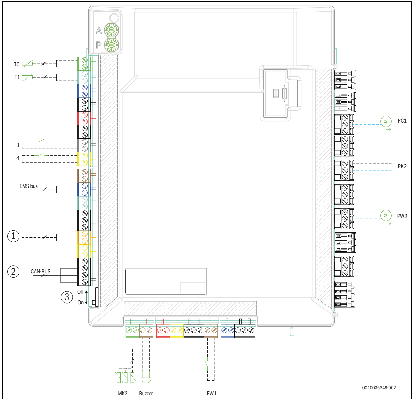
Bild 12 Inneenhetens installationsmodul
