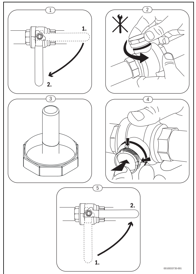
Bild 19 Rengöring av sil
