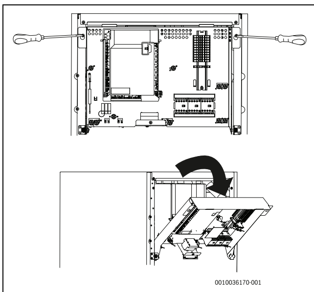
Bild 18 Luta kopplingsboxen
