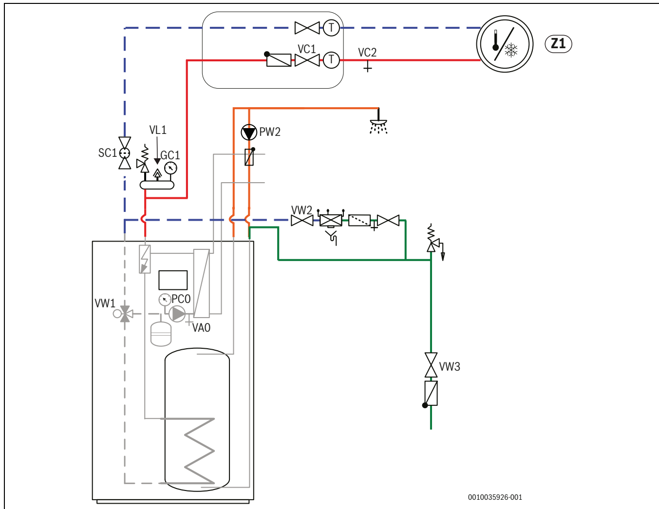
Bild 10 Inneenhet med integrerat eltilfskott och värmesystem
