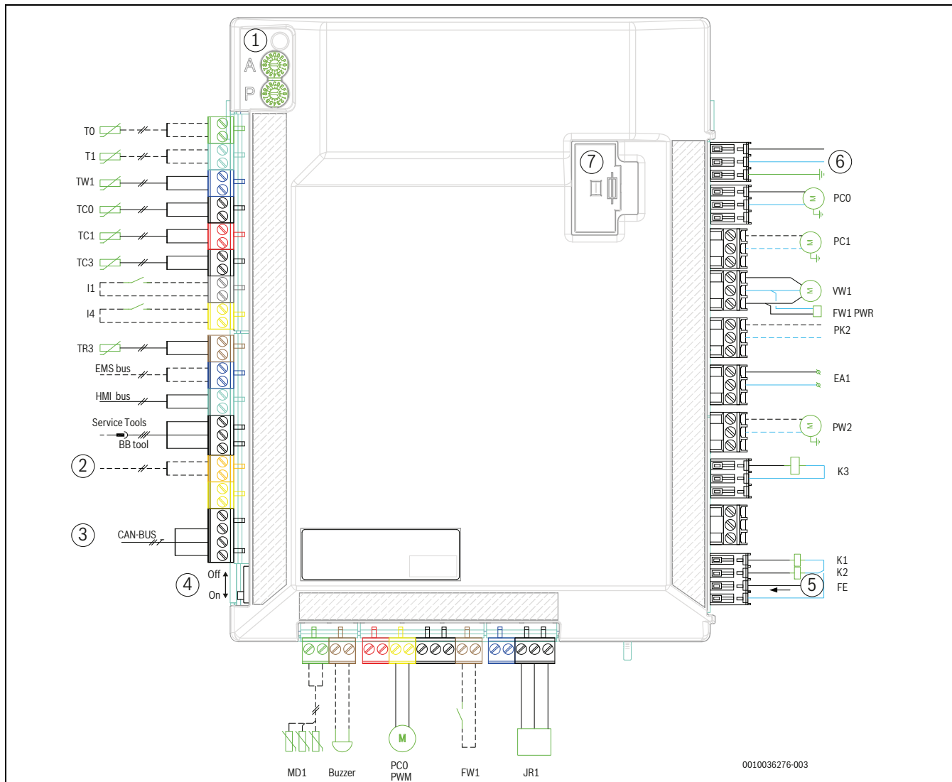
Bild 31 Inneenhetens installationsmodul
