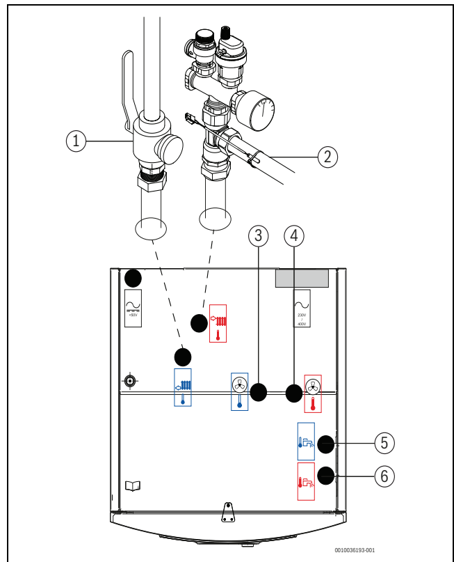
Bild 9 Inneenhetens anslutningar till värmesystemet och varmvattnet
