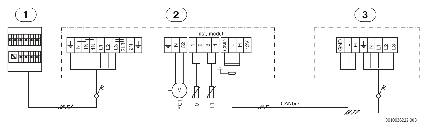
Bild 35 Kopplingsschema 9 kW 400 V 3 N~, alternativ koppling
