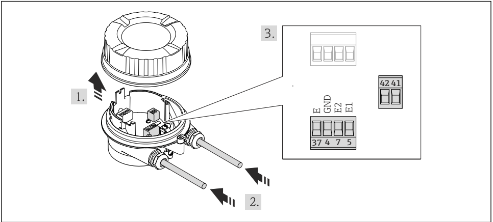
11 Sensor: anslutningsmodul
