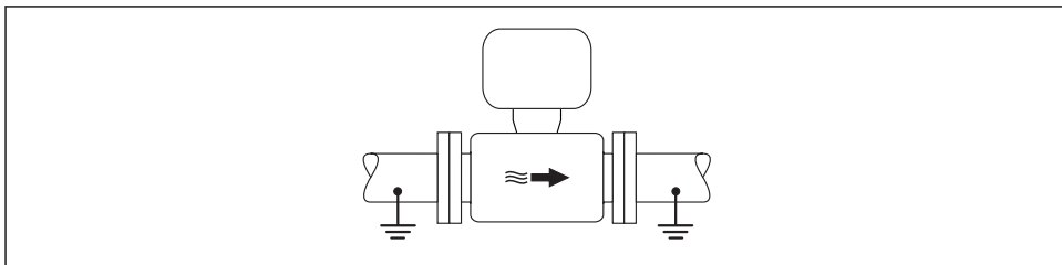
12 Potentialutjämning via mättröret
