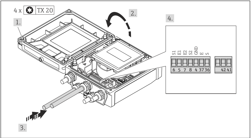
10 Transmitter: huvudelektronikmodul med plintar
