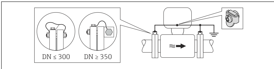
13 Potentialutjämning via jordanslutning och rörfänsar
