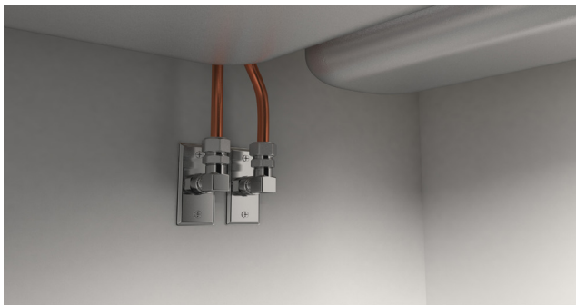
När genomföring av LK PE-X och PAL Universälror RiR utan väggdosa skall ansluta till t.ex. köks- eller tvättställsblandare, skall vinkeln i övergång mellan LK PE-X–LK PAL rör och blandarens anslutningsrör fixeras. Detta sker förslagsvis med väggbrička försedd med gänganslutning.
