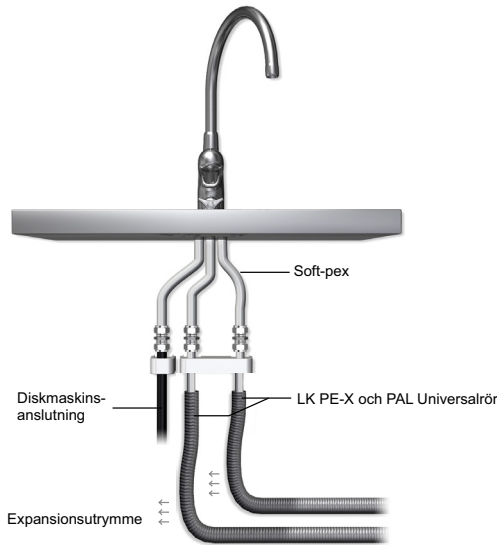
Godtagbar lösning vid installation av köksblandare med Soft-pex med LK PE-X och PAL Universälror RiR.
