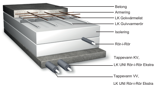
Förläggning av Rör-i-Rör i betongplatta med golvvärme.
