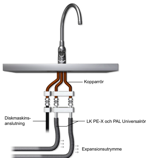
Godtagbar lösning vid installation av köksblandare med anslutningsrör av koppars med LK PE-X och PAL Universalrör RiR.
