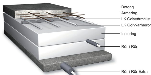
Förläggning av Rör-i-Rör i betongplatta med golvvärme. Rördragning av LK PE-X och LK PAL-rör till köksblandare
