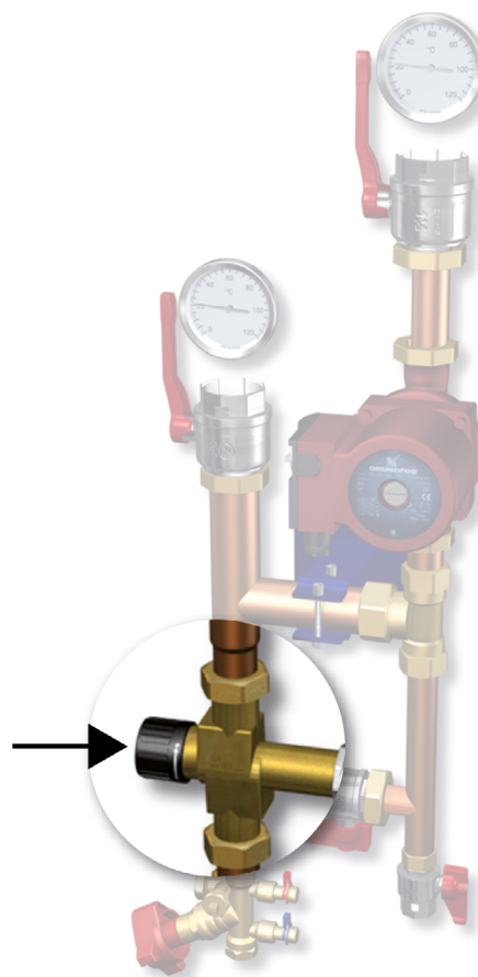
LK Shunt 2/3. Gänga av handratten och ersätt den med ventilställdonet.
