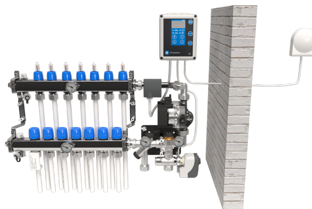
Monteringsexempel med LK Styr v.3 monterad på LK Fördelarshunt VS2
