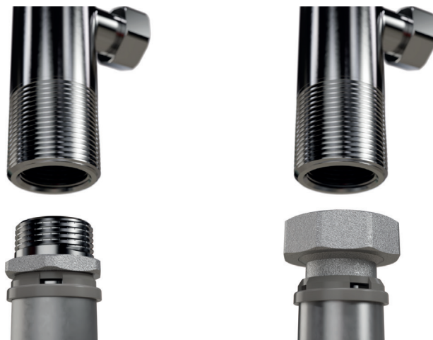
Bilden visar invändig och utvärdig gänga för anslutning av kopplingar mot LK PVK.
