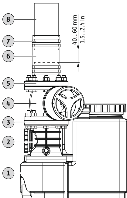
Fig. 3: Montera tryckanslutningen
