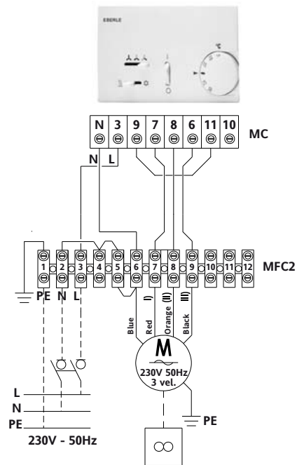
T2T-FUTURA Termostatazione sul ventilatore T2T-FUTURA Thermostatic control on the fan
