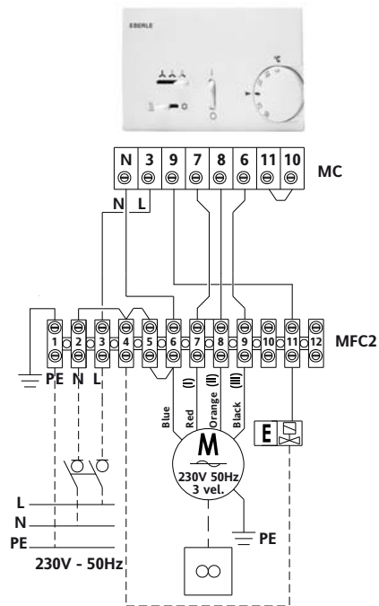
T2T-FUTURA Termostatazione sulla valvola e funzionamento continuo del ventilatore T2T-FUTURA Thermostatic control on the valve and continuous fan operation
