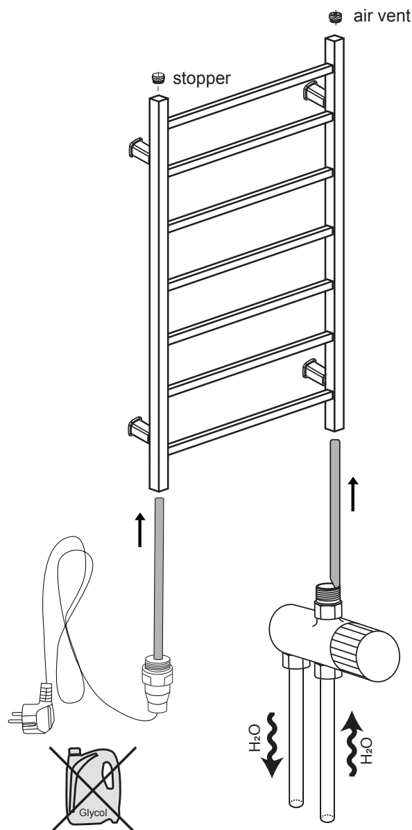
D4 (UK) Combination of electrics system and closed heating (SE) Kombination av elpatron och slutet värmesystem
