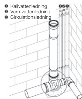
Installationsexempel kombinationsgrenrör (FIGUR 32)
