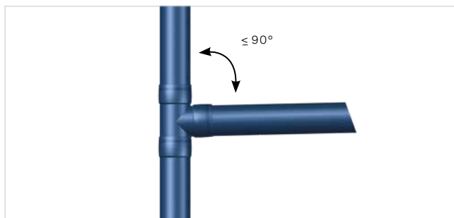
Anslutning till stående ledning endast med grenrör med max. 90° vinkel.
