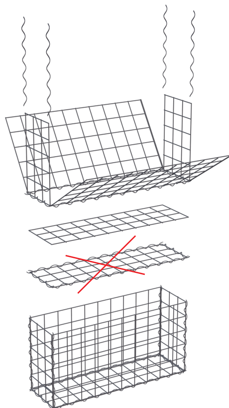
EXEMPEL: MONTERING AV GABIONKORGAR STAPLADE ÖVER VARANDRA
