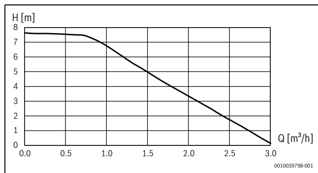
Bild 26 Kapacitetskurva för den primära cirkulationspumpen (PC0)
