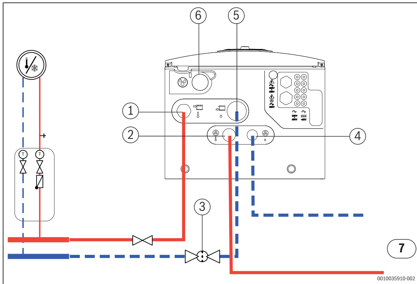
Bild 8 Anslutning av en inomhusenhet med ett integrerat eltillskott till en utomhusenhet och ett värmesystem
