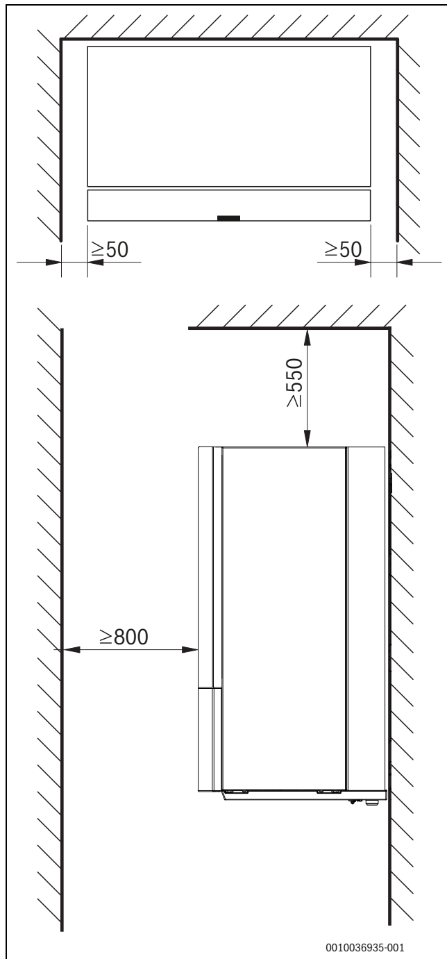
Bild 4 Minimiavstånd (mm)
