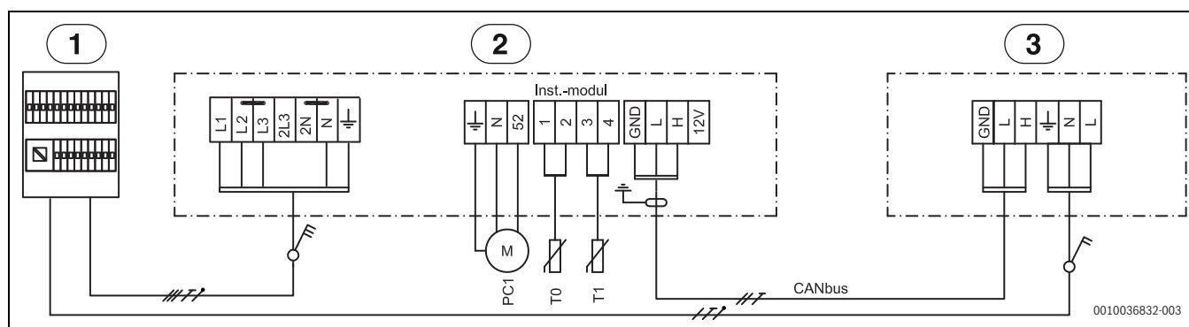
Bild 37 Kopplingsschema 9 kW 400 V 3N~
