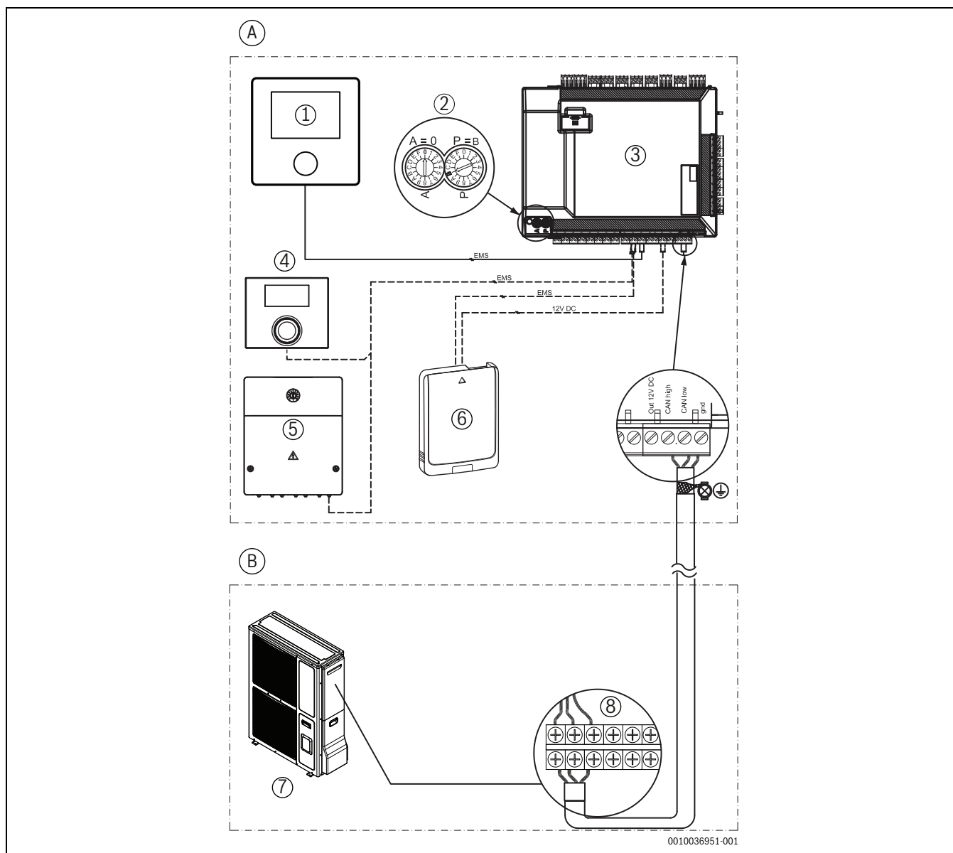
Bild 35 CAN- och EMS-anslutningar
