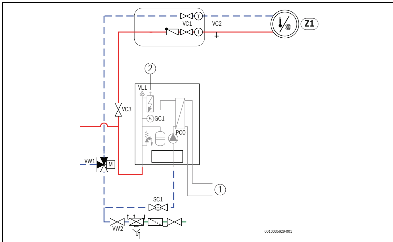
Bild 9 Inomhusenhet med integrerat eltilskott och värmesystem
