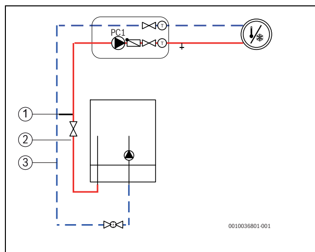
Bild 27 Inneenhet med värmekrets och bypassledning
