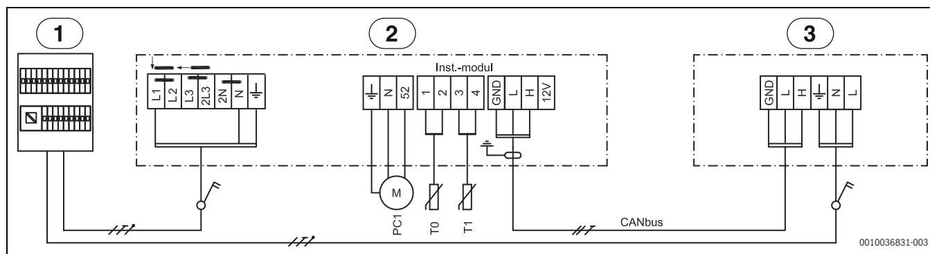
Bild 36 Kopplingsschema 9 kW 230 V~
