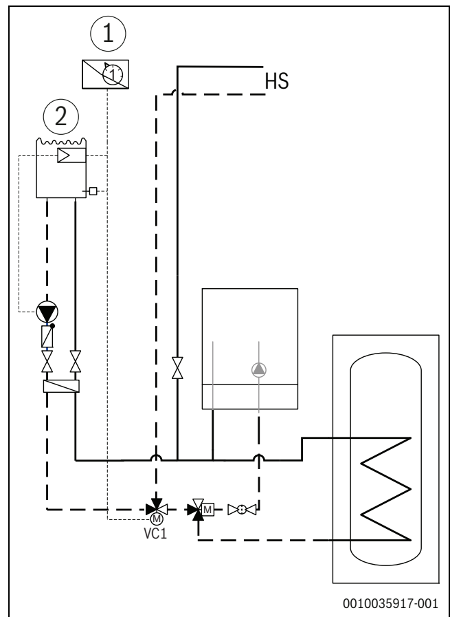
Bild 24 Poolinstallation exempelbild
