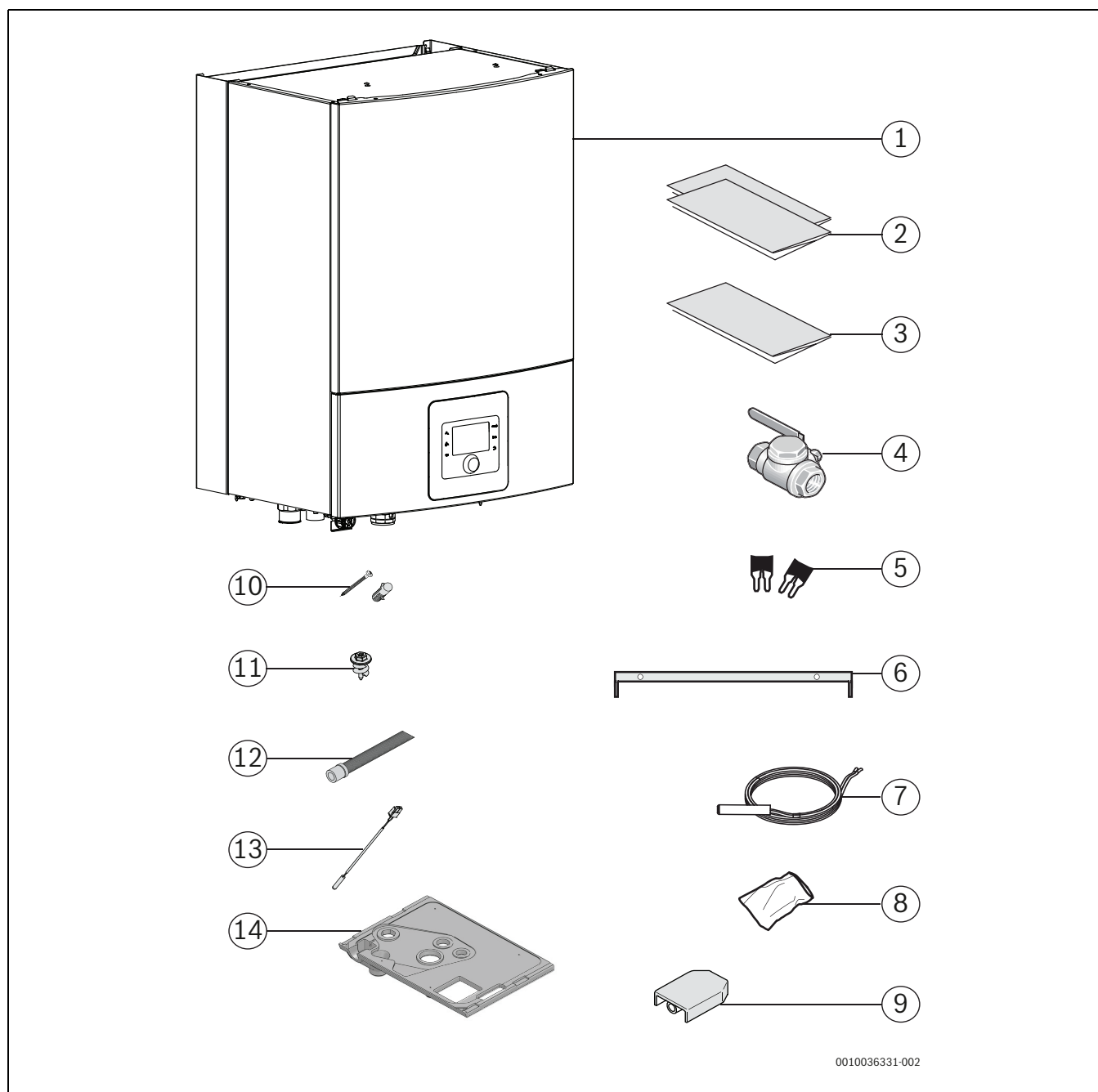
Bild 2 Leveransinnehåll
