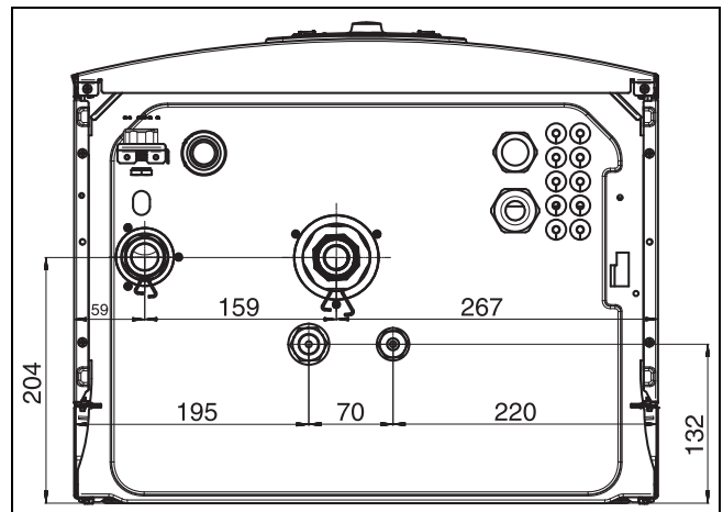
Bild 5 Mått och anslutningar (vy utan dropptrång)
