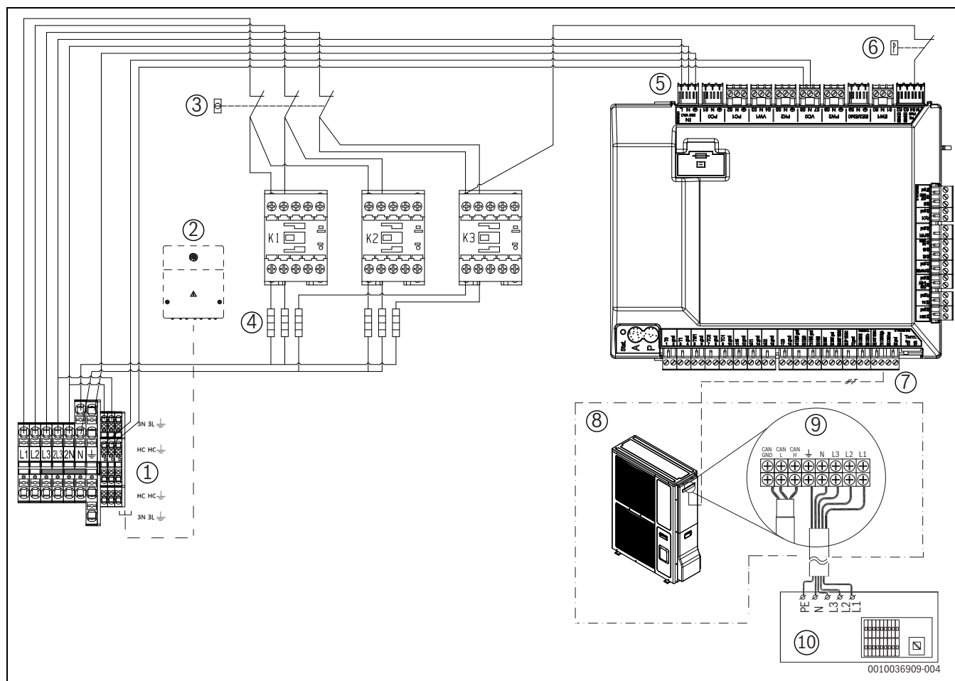
Bild 40 400 V 3N~ inomhusenhet med 400 V 3N~ utomhusenhet
