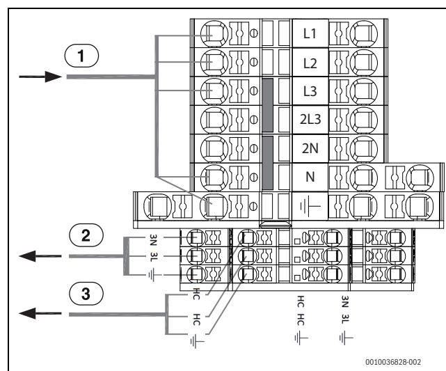
Bild 14 Anslutningsplintar för elanslutning, 9 kW 400 V 3N~
