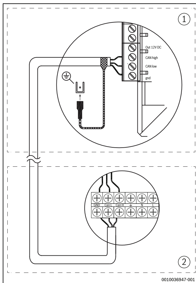
Bild 12 CAN-BUS-anlutning
