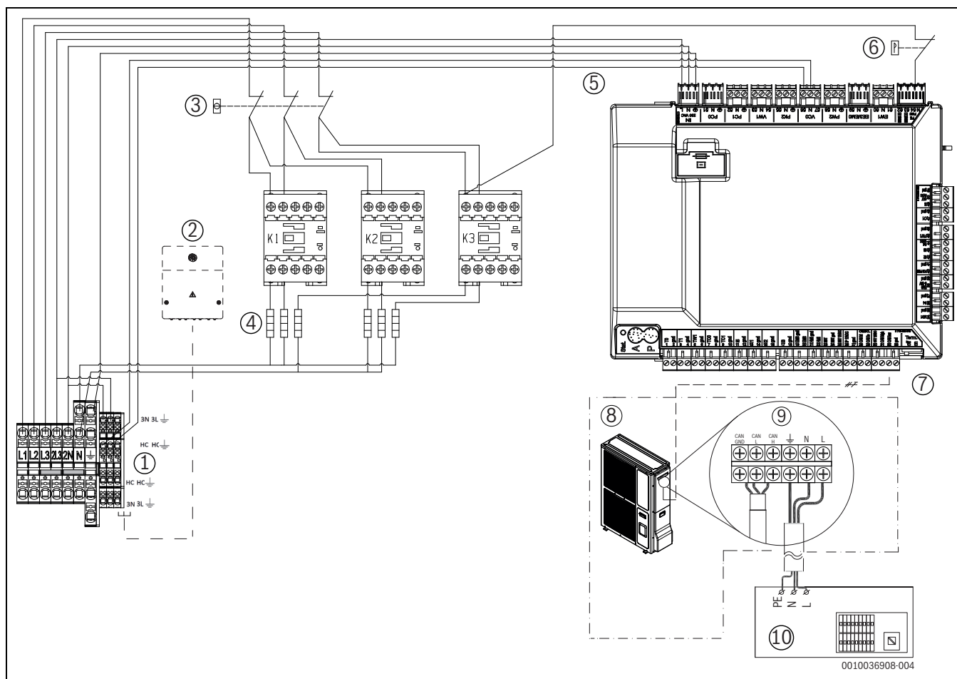
Bild 39 400 V 3N~ inomhusenhet med 230 V~ utomhusenhet
