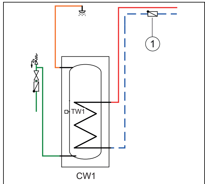
Bild 18 Varmvattenberedare
