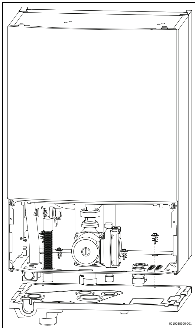
Bild 7 Montera dropptråget
