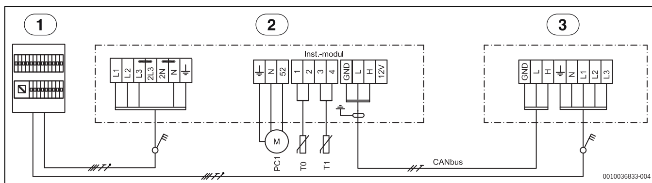
Bild 38 Kopplingsschema 9 kW 400 V 3N~
