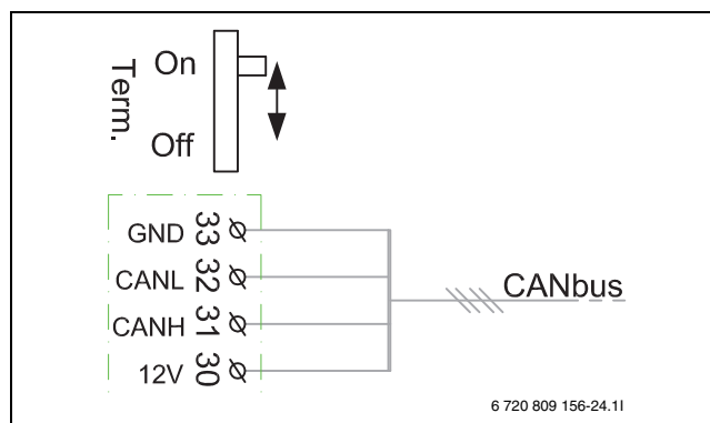
Bild 10 Terminering CAN-BUS
