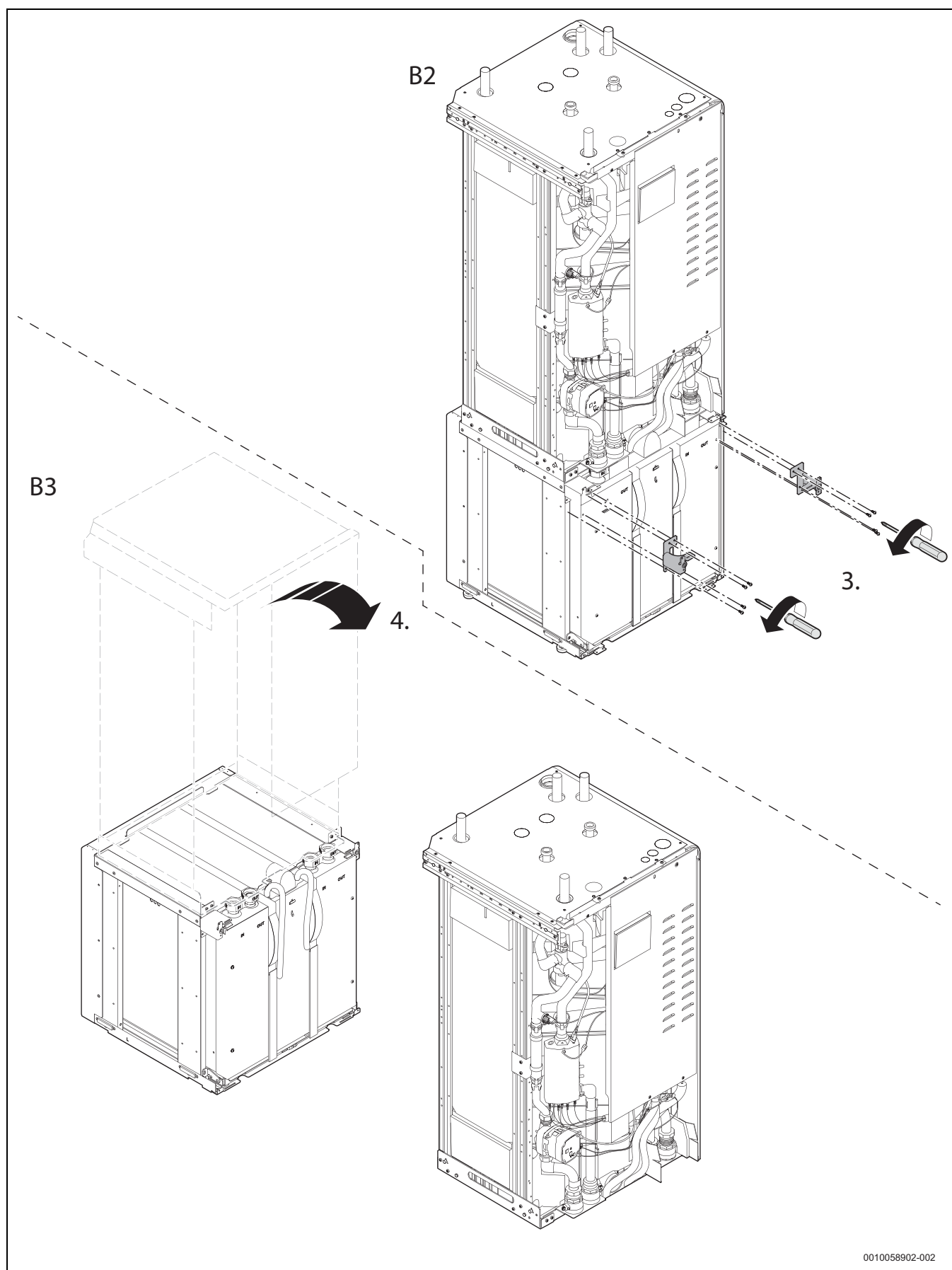
Bild 13 Delning värmepump
