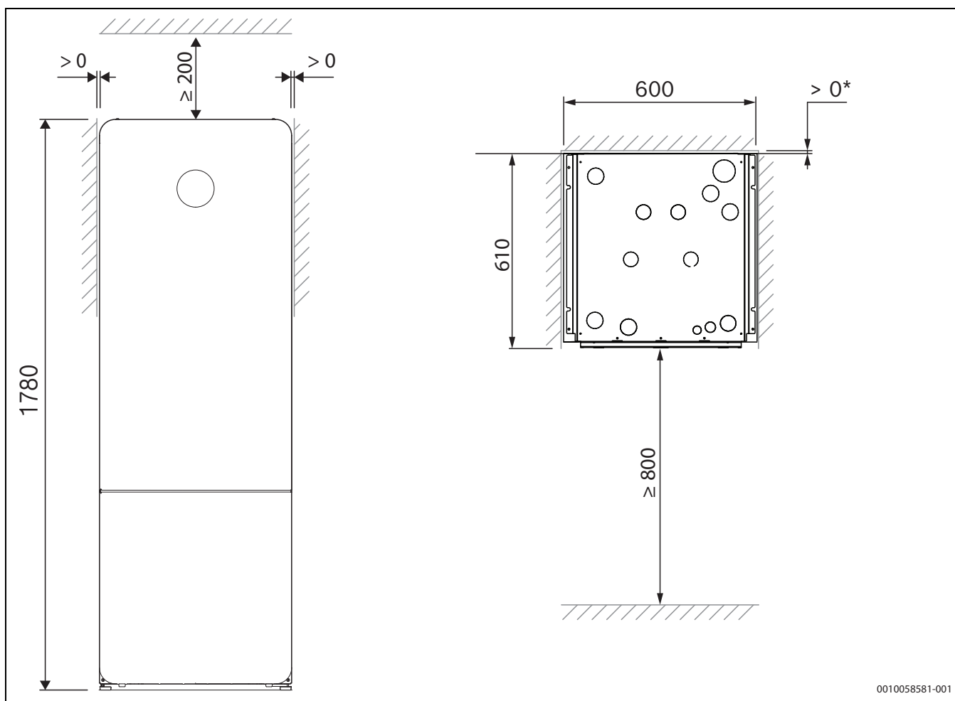
Bild 2 Mått och minimiavstånd
