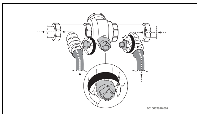
Bild 48 Påfyllnadssats i påfyllningsläge
