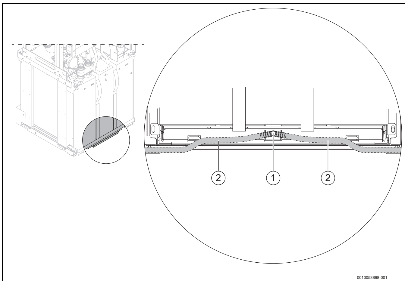
Bild 42 Ansluta dräneringsslang
