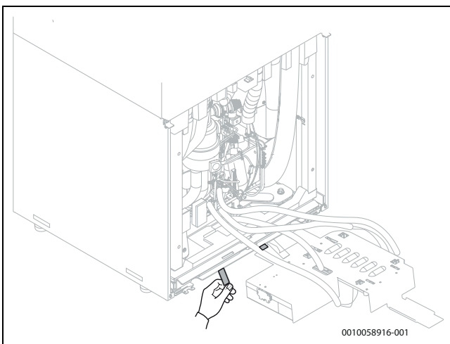
Bild 22 Ta bort markeringsremmarna
