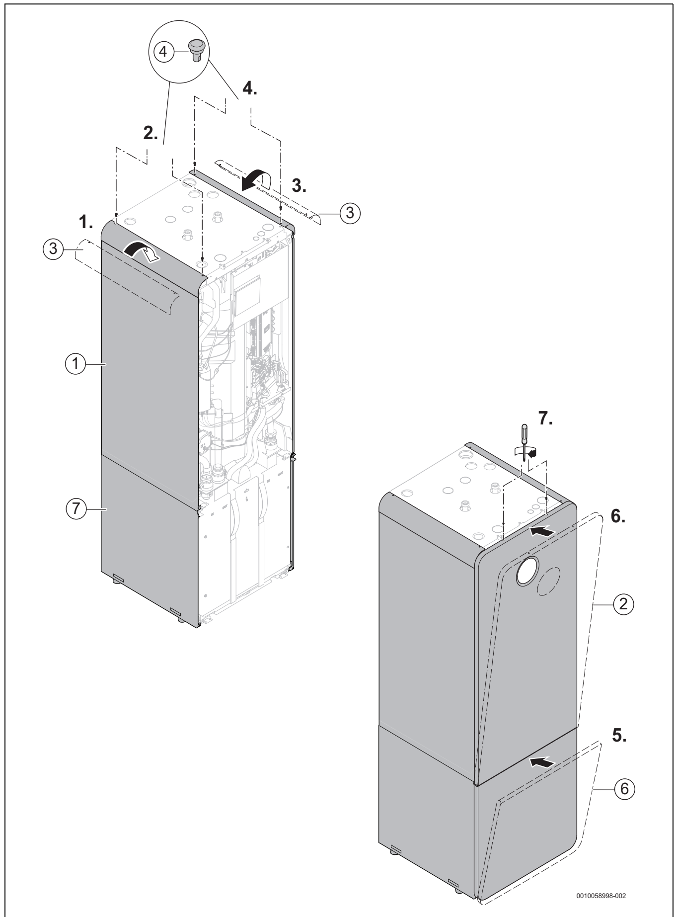
Bild 8 Montering av design-kit
