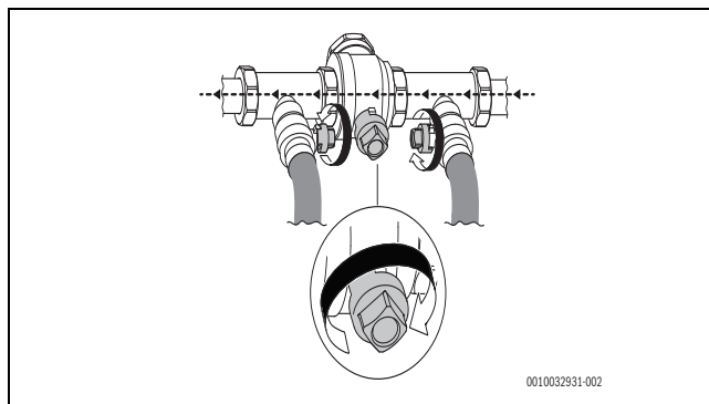
Bild 52 Påfyllnadssats i normalläge
