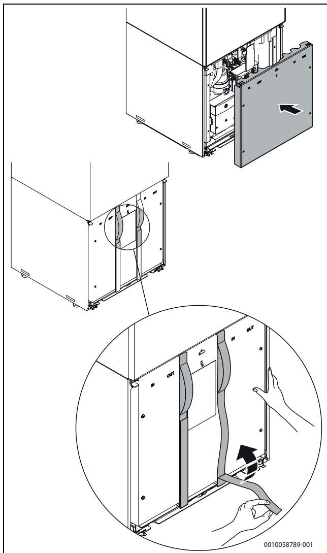
Bild 26 Sätt tillbaka frontplåten
