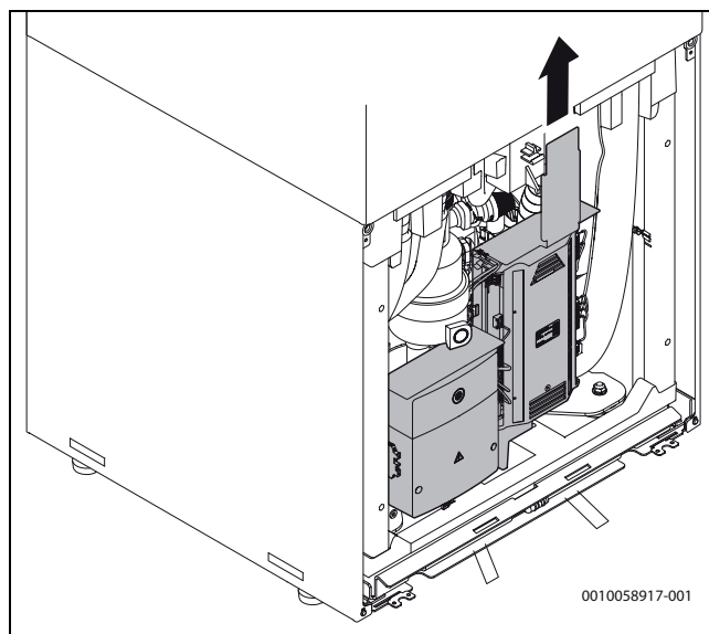
Bild 20 Ta bort elpanelen
