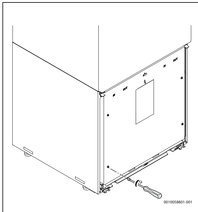
Bild 27 Installera och dra åt de 4 skruvarna
