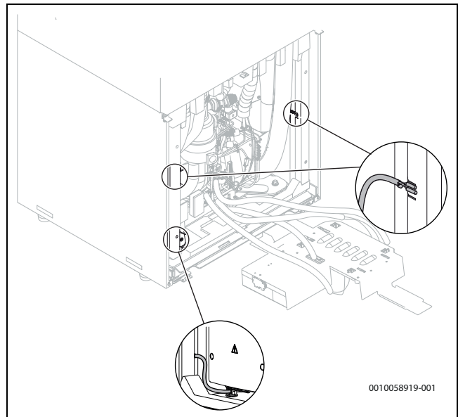
Bild 24 Kontrollera slang och jordningskabel
