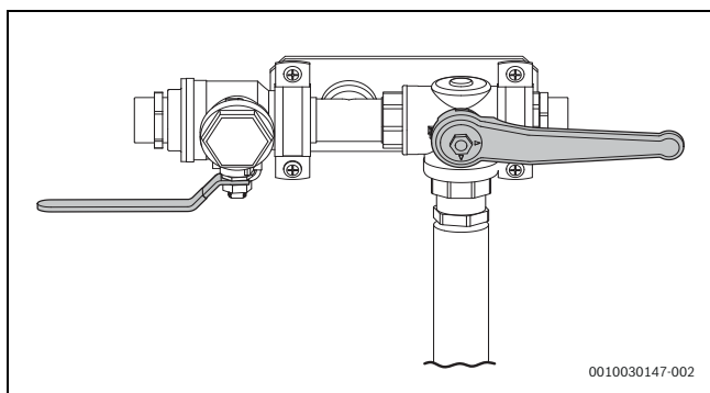
Bild 50 Påfyllnadsstation i påfyllningsläge
