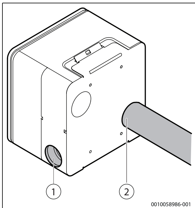
Bild 29 Inlopp och utlopp, fläktlåda
