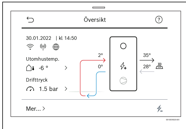
Bild 63 Översikt av värmepumpen
