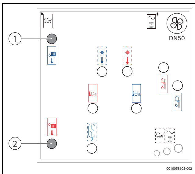
Bild 44 Anslutning av värmepumpen till värmesystemet
