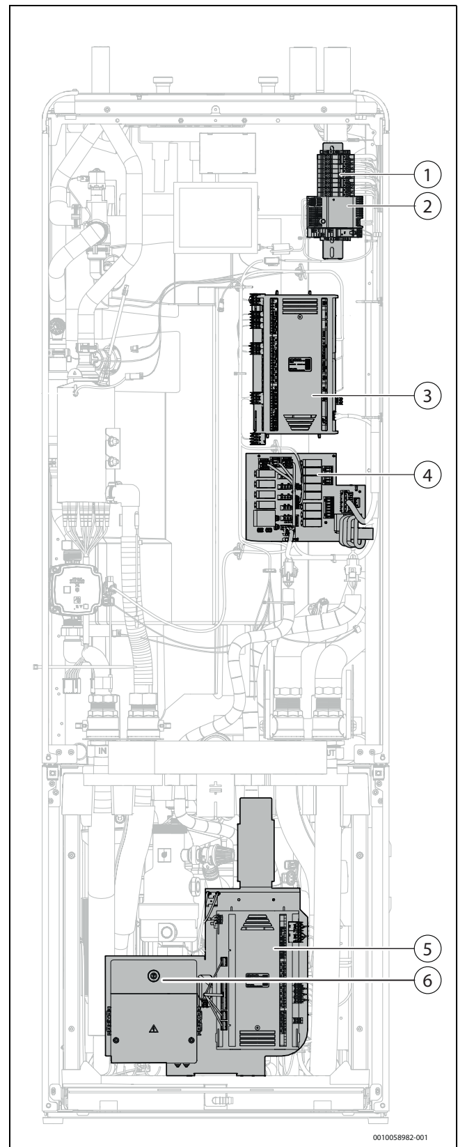
Bild 54 Elektriska komponenter och reglercentraler
