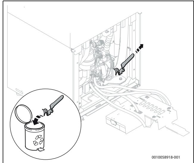
Bild 23 Ta bort transportfästet
