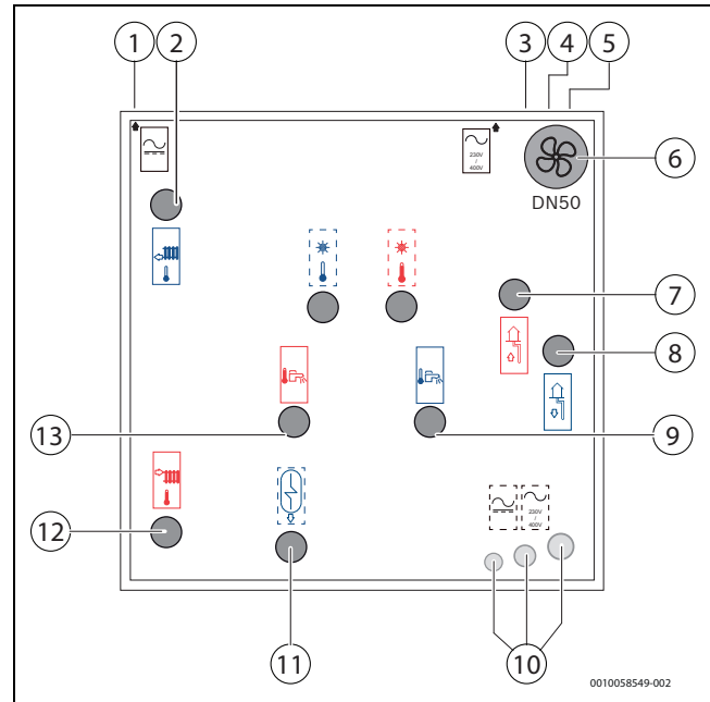
Bild 5 Anslutningar värmepump, takvy
