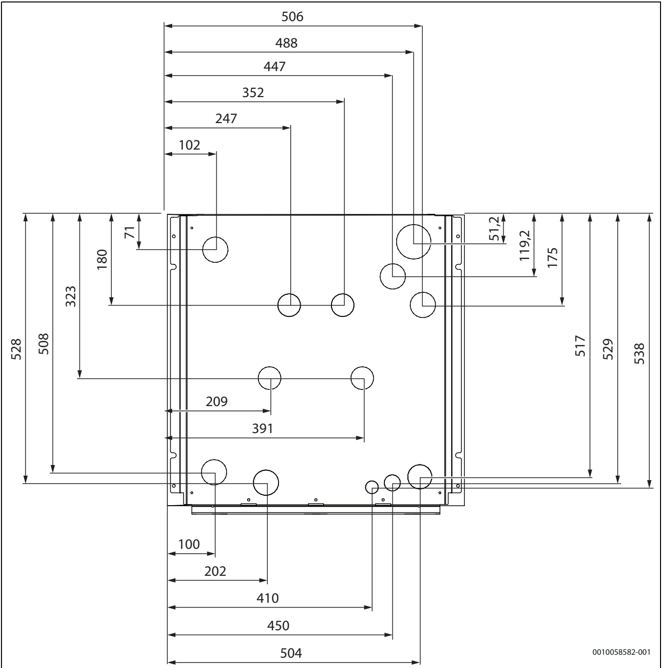
Bild 3 Mått anslutningar, takvy
