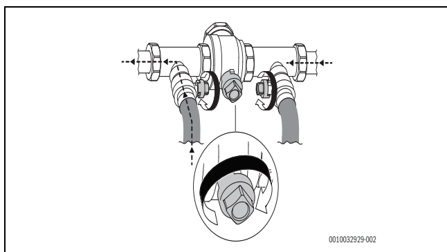
Bild 51 Påfyllnadssats i tryckhöjningsläge
