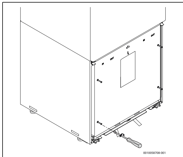
Bild 18 Lossa de 4 skruvarna
