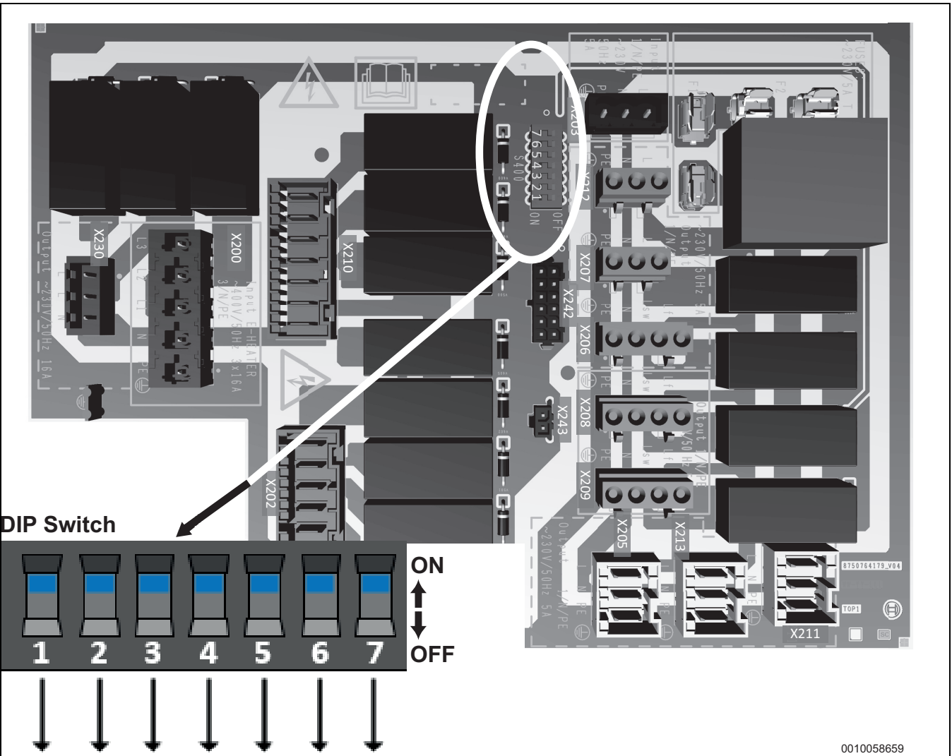
Bild 62 Begränsning av elektrisk extra värmekälla
