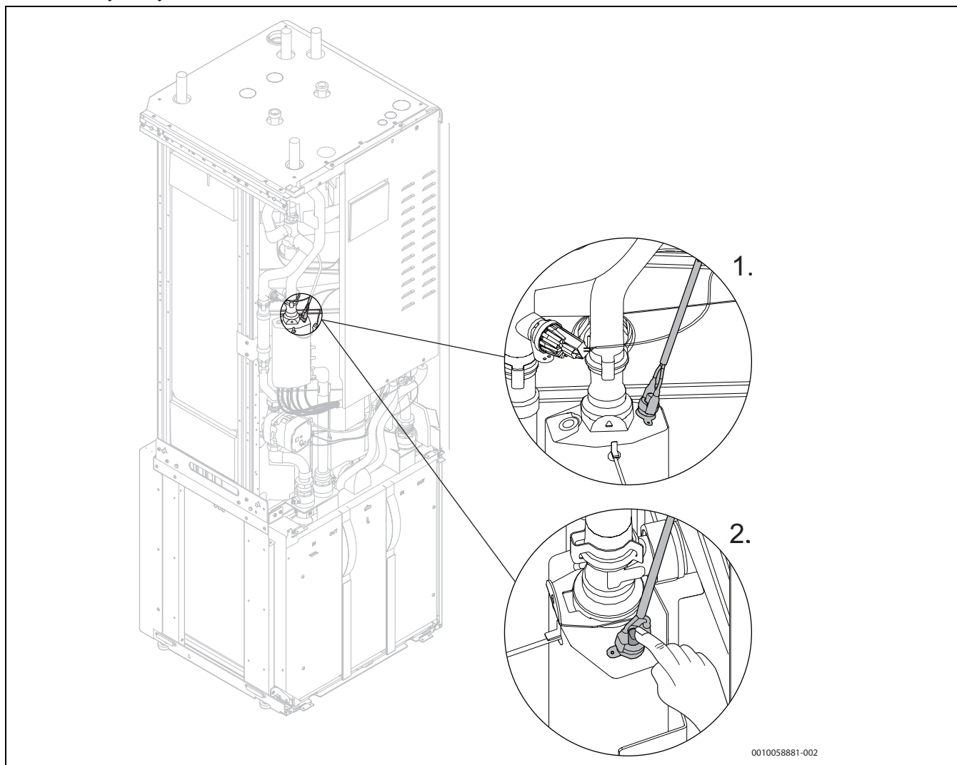
Bild 65 Återställa överhettningsskyddet
