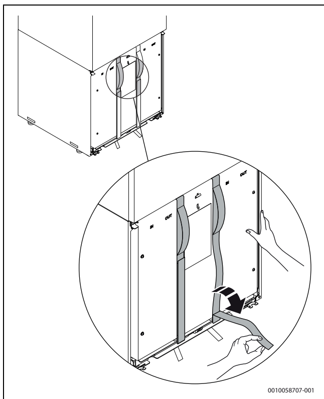
Bild 17 Lossa remmarna
