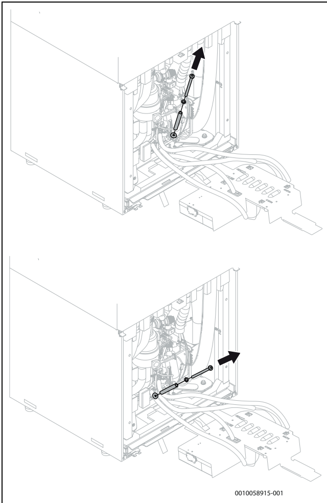
Bild 21 Ta bort skruvarna som håller fästet
