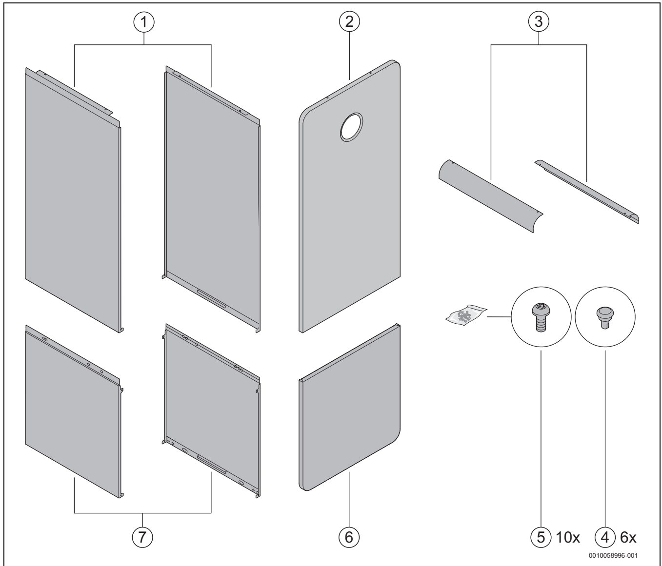
Bild 6 Montering av design-kit
