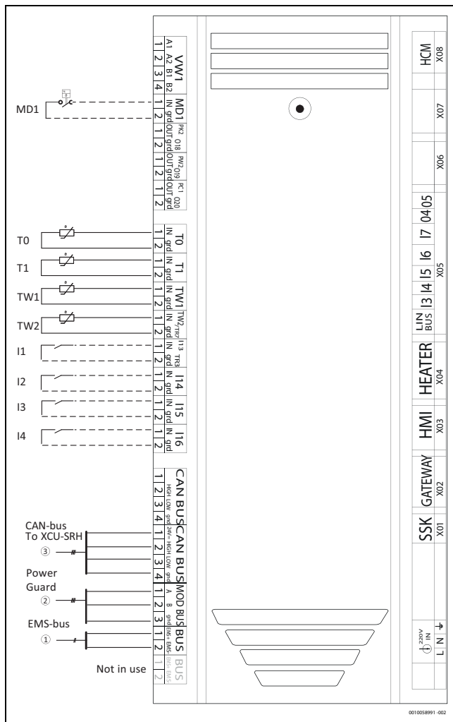
Bild 58 Anslutningsmöjligheter XCU-THH
