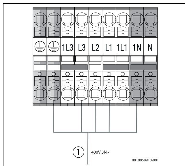
Bild 56 Elmatning standard från fabrik (6 kW, 8 kW, 13 kW, 17 kW)
