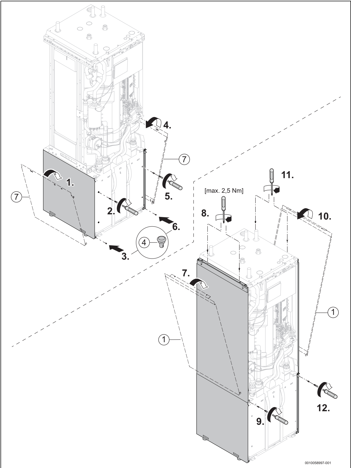
Bild 7 Montering av design-kit
