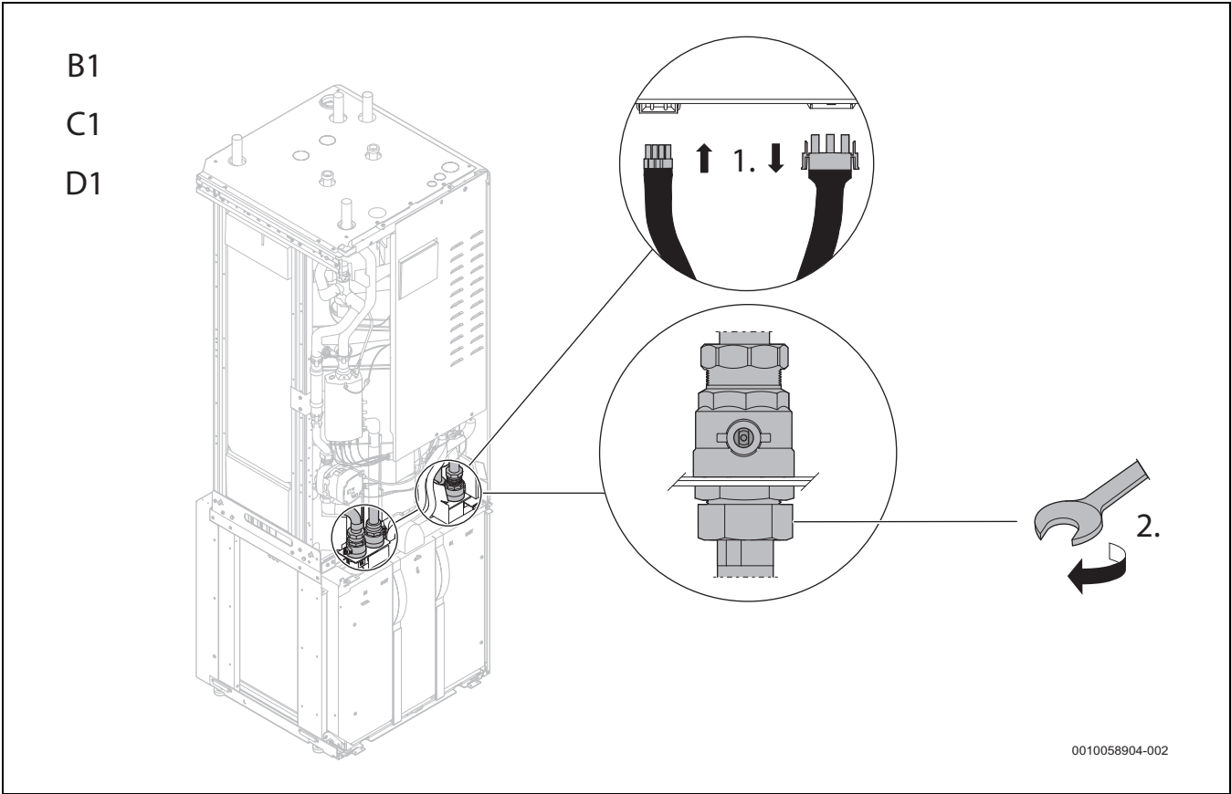
Bild 12 Delning värmepump
