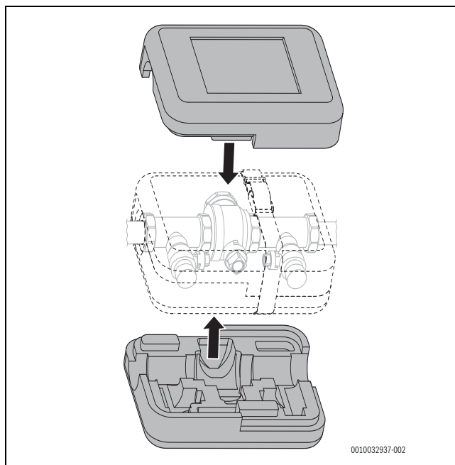
Bild 53 Isolering av påfyllnadssats
