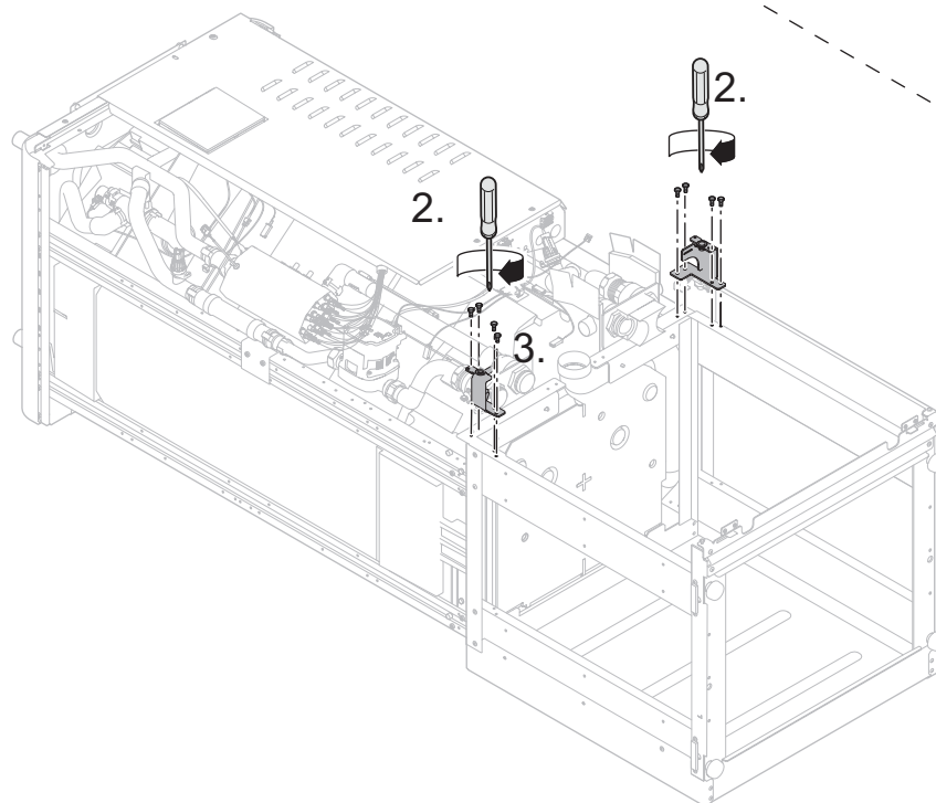
Bild 15 Delning värmepump
