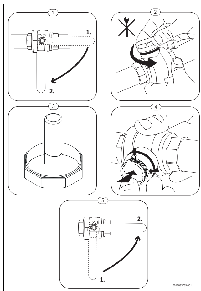
Bild 64 Rengöring av sil
