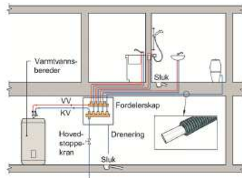
Fig. 1 Prinsippskisse for rør-i-rør-system
