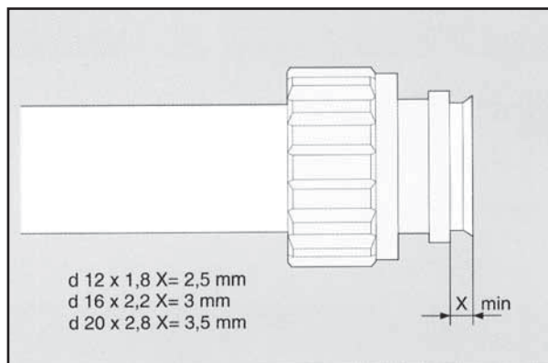
Kontroll av monteringsresultat: konflänsen för PEX-röret på en korrekt monterad konkoppling måste minst ha de i figuren angivna X-måtten
