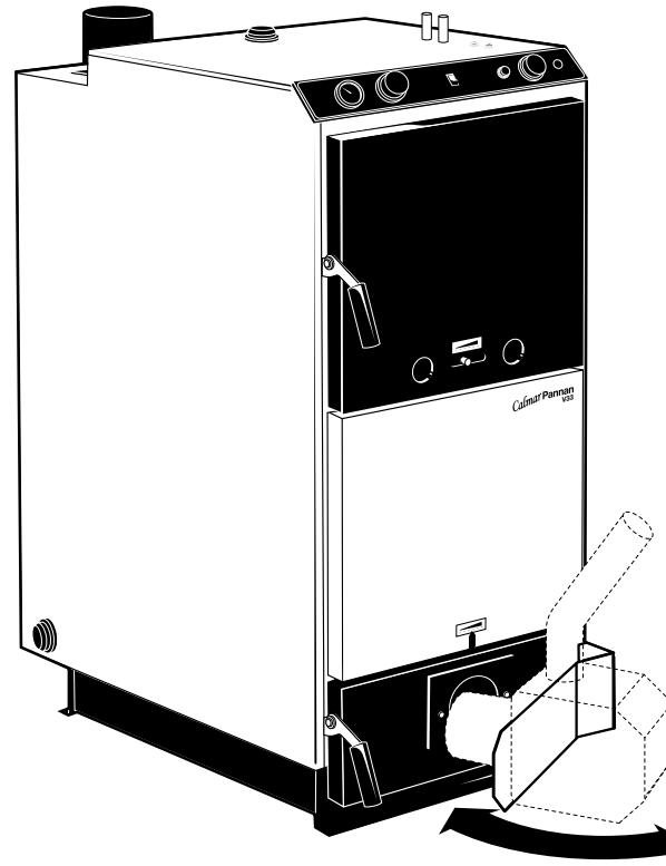
7.2 Principinstallation av oljebrännare monterad
