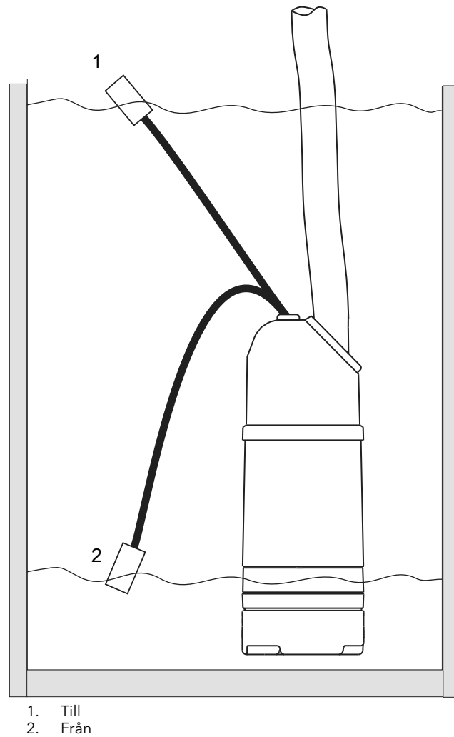
Figur 1: Nivåregulatorns funktion
