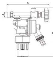
STBA 400 Med slanganslutning och avstängningsventil
