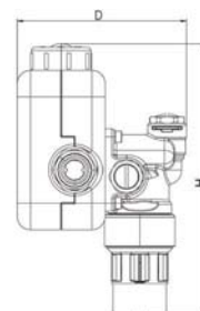
STBA 600 Standardutförande med inbyggd reduceringsventil och manometer
