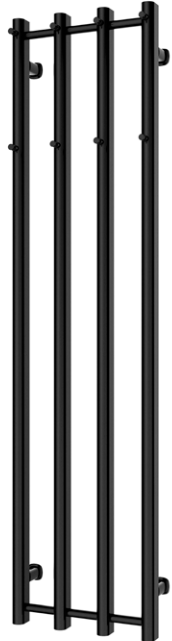
4-rör, matt svart 351 x 1 400 mm (b x h) Effekt: 375 W Art nr 873 02 48
