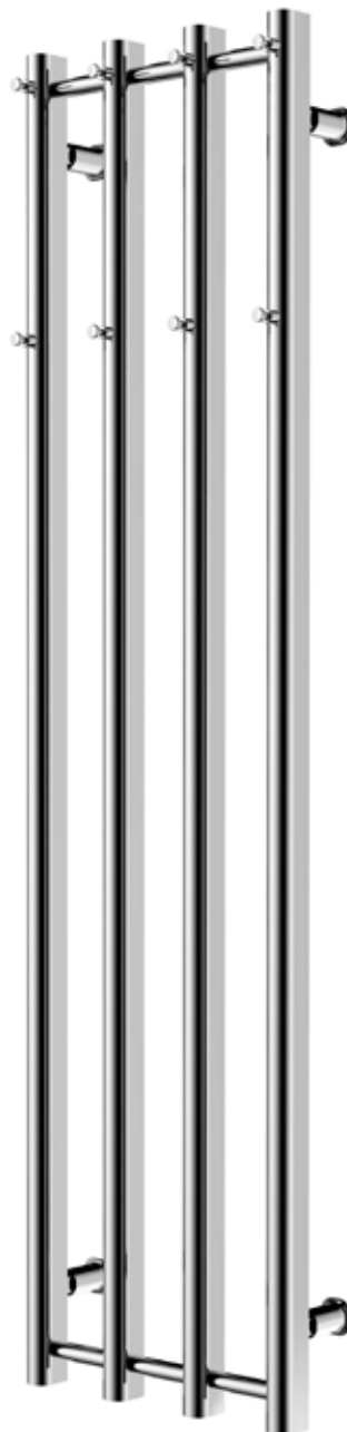
4-rör, krom 351 x 1 400 mm (b x h) Effekt: 290 W Art nr 876 05 29
