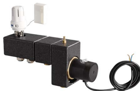
Uponor Fluvia T Push-12 TH-X. Rumsgivare med kapillärrör och känselkropp.
