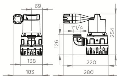
Sanisub 400
