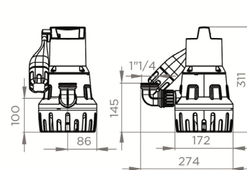
Sanisub 800
