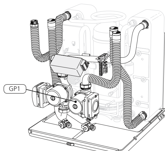
Pumpen är ställbar, flödet kan justeras i meny 5.1.11. Bilden visar kyldele F1155-16.
