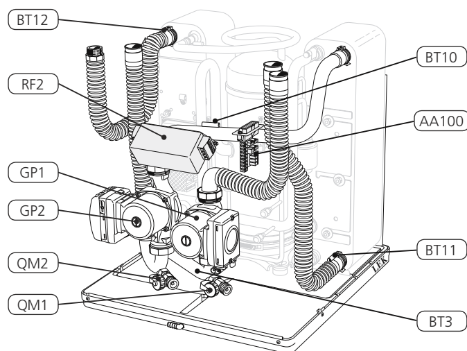
Komponentplacering i kyladel F1155-16
