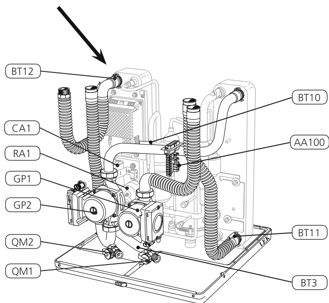
Komponentplacering i kyladel F1155-6
