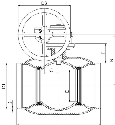
DN 100-500
