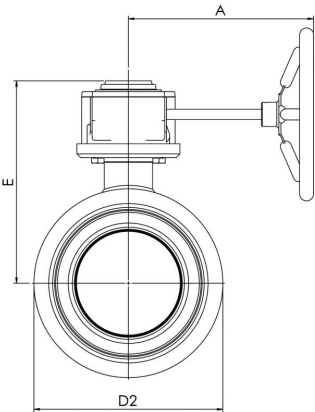
DN 100-500
