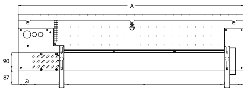
Ovanifrån
