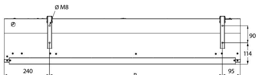
Baksida
