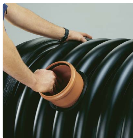
4. Montera anslutningsröret
