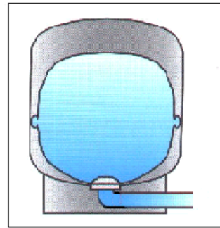
Pumpen stannar - membranhydroforen är fylld med vatten
