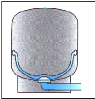
Pumpen startar innan membranhydroforen är helt tömd på vatten
