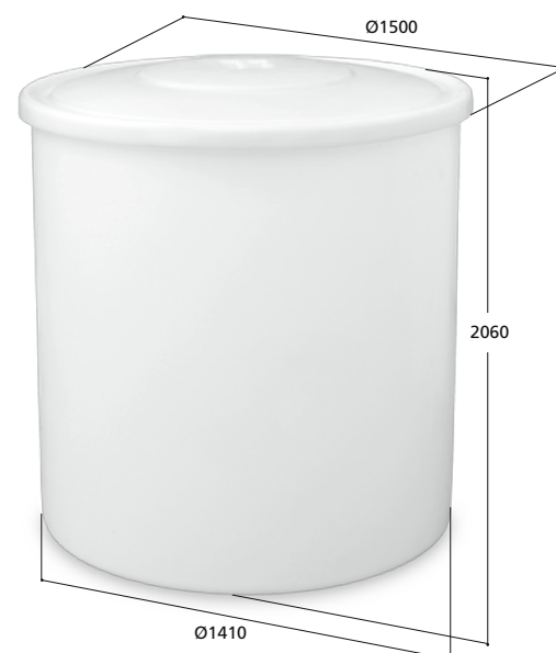
Volym 3000 liter Art. nr 13000
