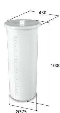
Volym 110 liter Art. nr 10110
