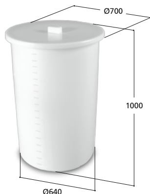
Volym 320 liter Art. nr 10320
