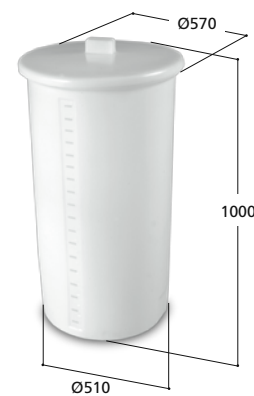
Volym 200 liter Art. nr 10200
