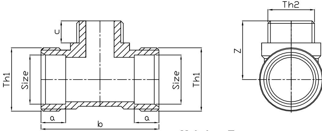
Male Iron Tee Cu x Cu x M
