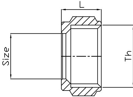
P163 Nut
