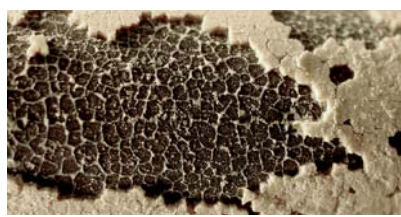
Kalkavlagring
