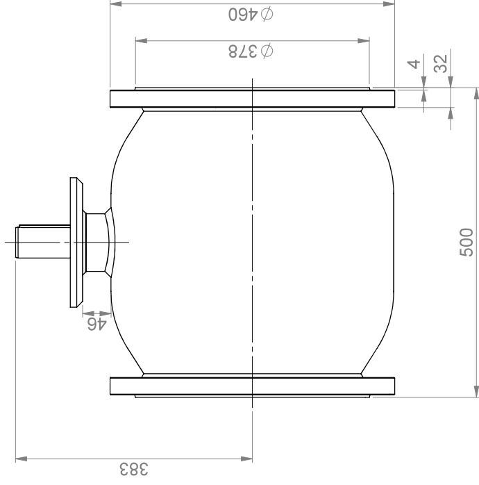
ISO 5211 Top Flange F16
