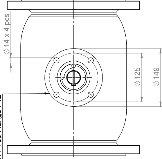
ISO 5211 Top Flange F12
