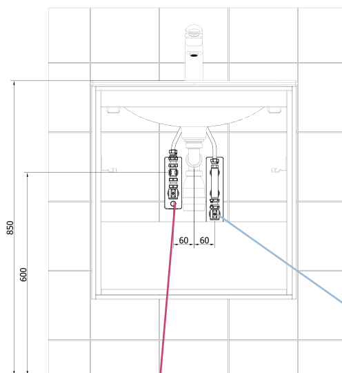
Installation bakom kommod
