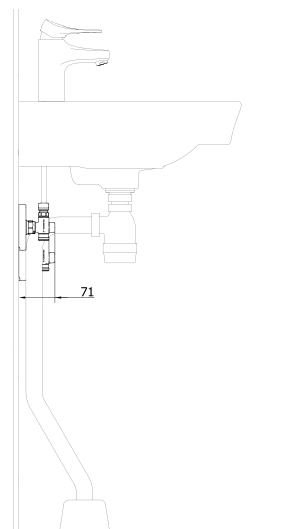
Installation under tvättställ
