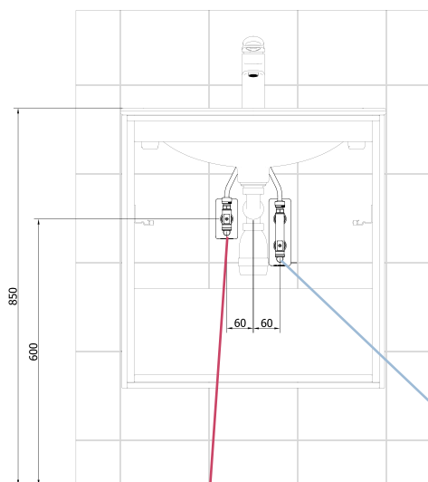
Installation bakom kommod
