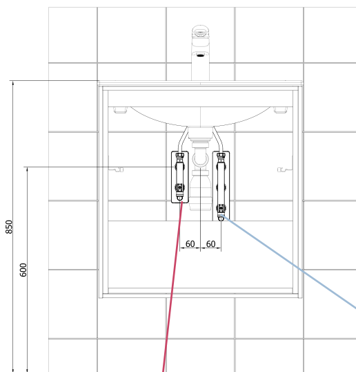
Installation bakom kommod
