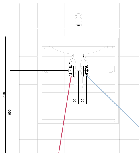
Installation bakom kommod
