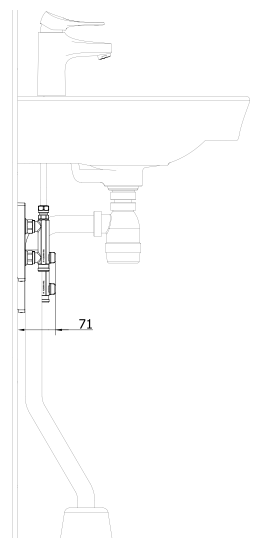
Installation från sidan
