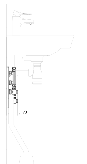
Installation från sidan
