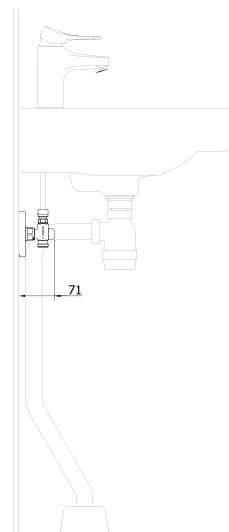
Installation under tvättställ
