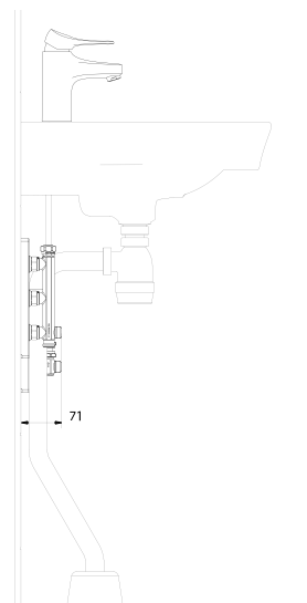
Installation från sidan
