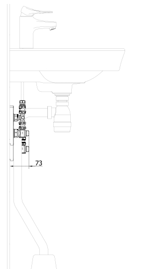
Installation från sidan
