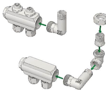
Montage av anslutningsrör till LK Minifördelare 2-kretsar.
